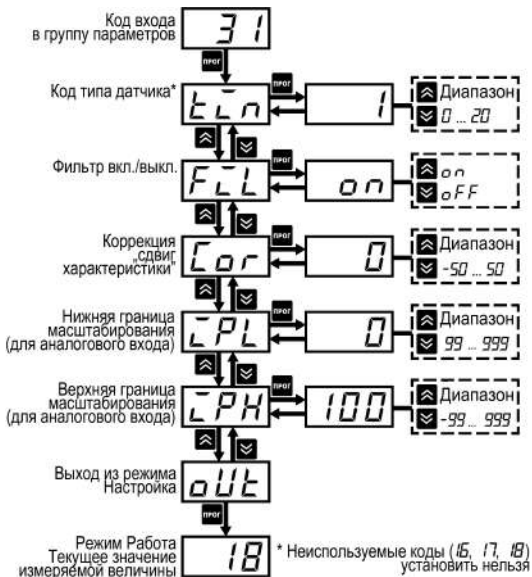
Рисунок 7.2 – Настройка параметров входа
