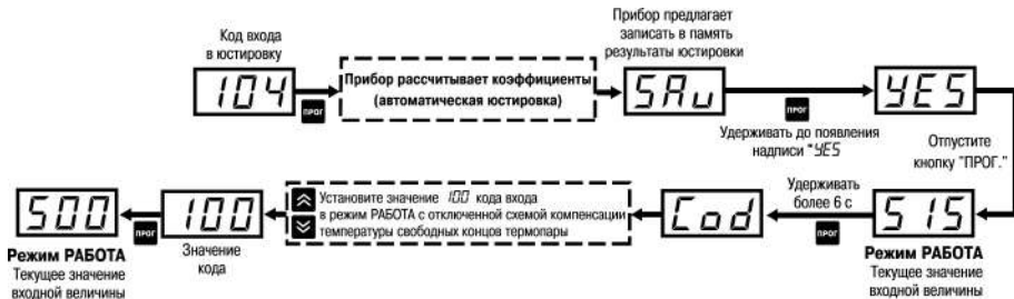
Рисунок 8.6 – Схема юстировки прибора с ТП
